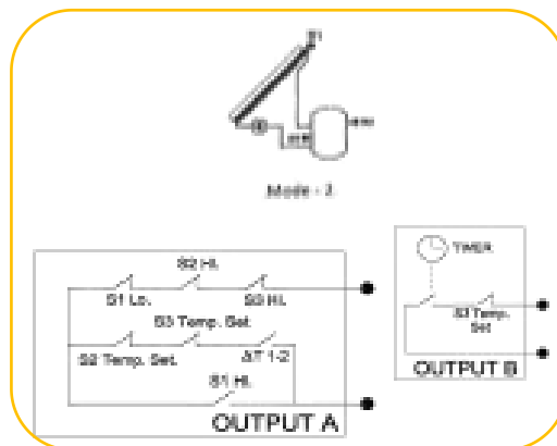
Εφαρμογή 2: 3 αισθητήρια με βοηθητική πηγή
